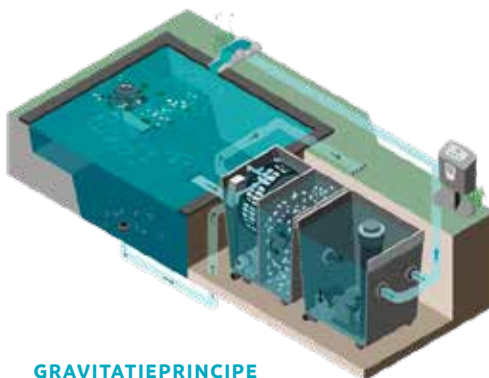
GRAVITATIEPRINCIPE
